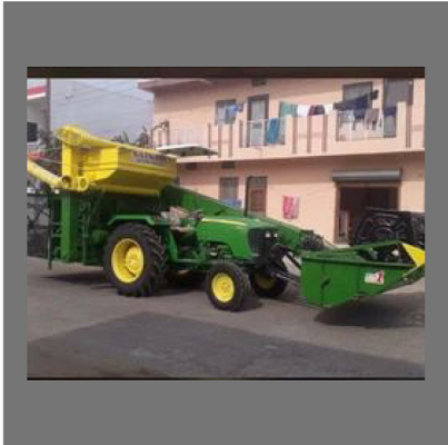
Mini Combine Harvester
